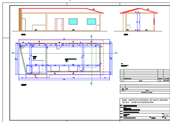
FIGURA 1 – PROJETO ARQUITETÔNICO DA SALA DE INFORMÁTICA
